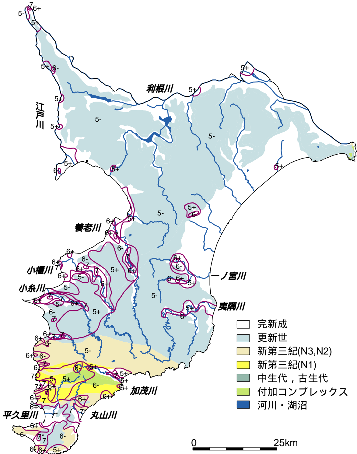
図4 震度分布と表層地質との比較
