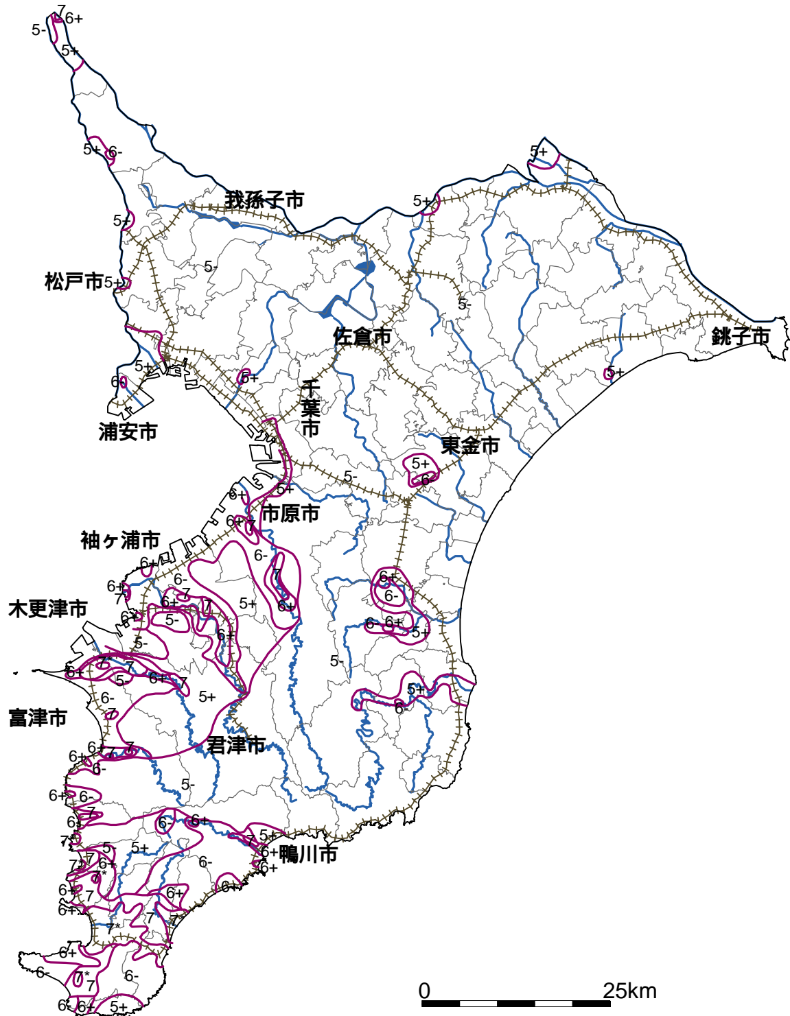
図5 最近の市区町村地図の上に描いた関東地震の震度分布
