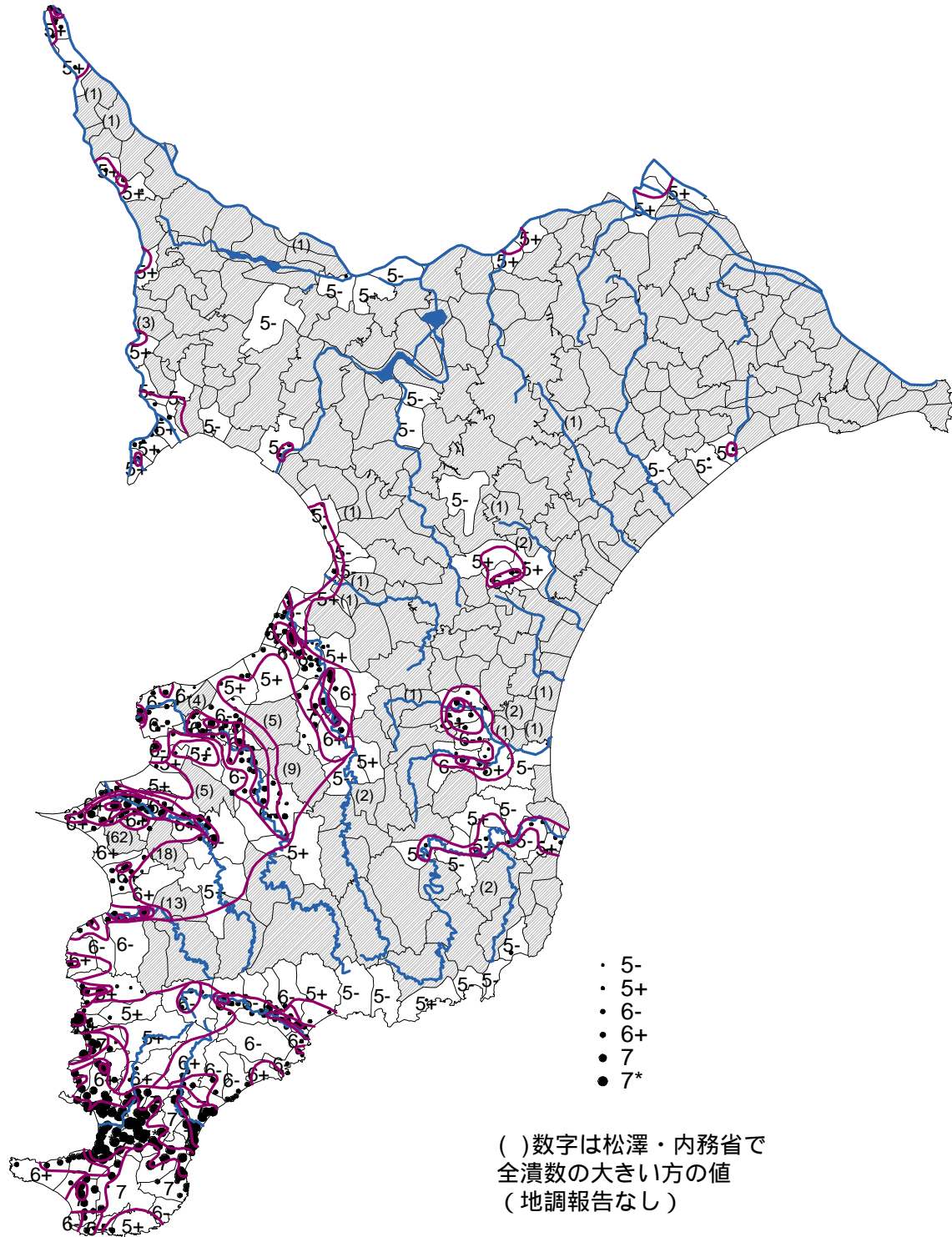
図3 千葉県全体の震度の評価値と震度の境目コンター
