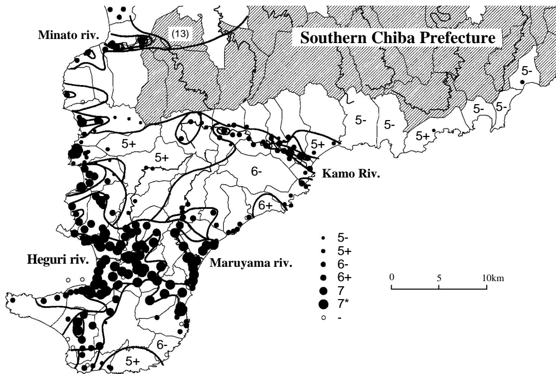
図2 千葉県南部の震度の評価値と震度の境目コンター
