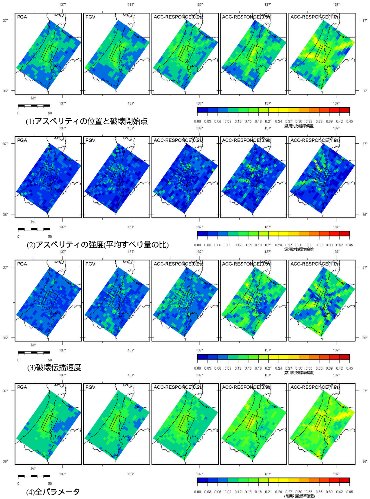
図 10 バラツキの対数標準偏差の空間分布(統計的グリーン関数法)
