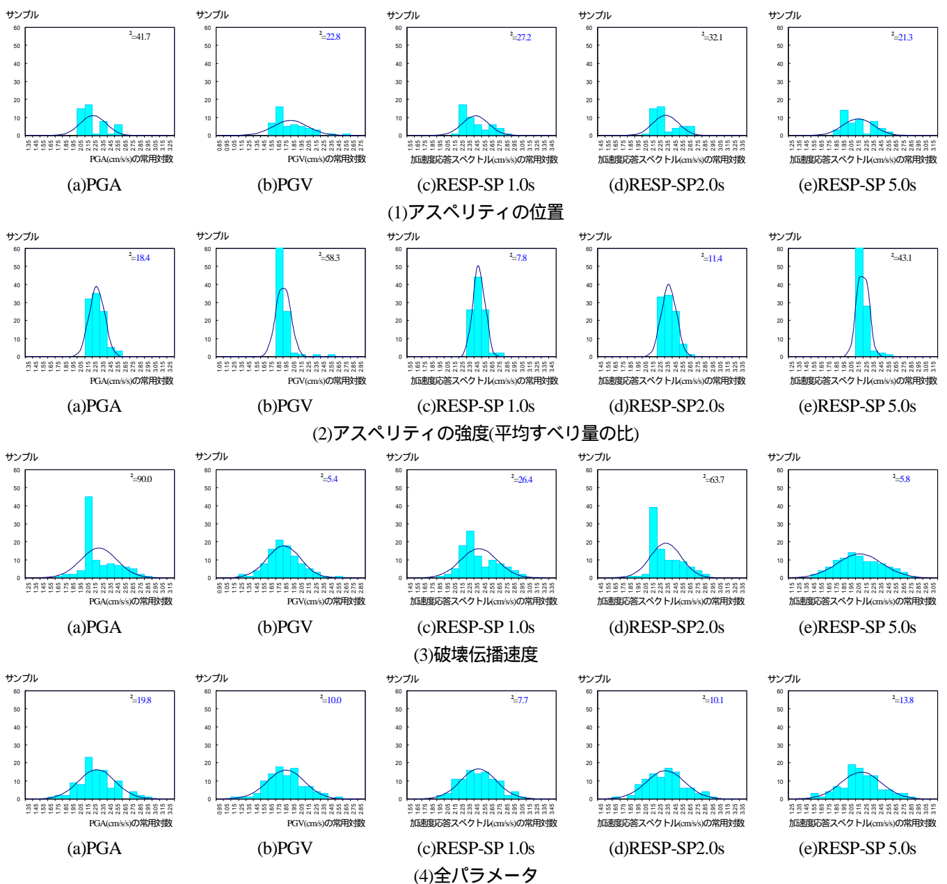
図8 強震動予測結果のヒストグラム(差分法)
