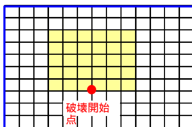
図3 アスペリティの位置と破壊開始点
