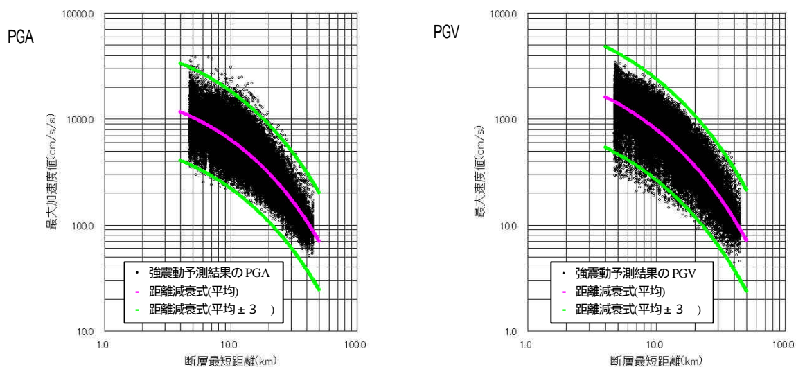
図14 距離減衰式との比較
