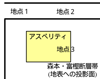
図4 パイロットポイント
