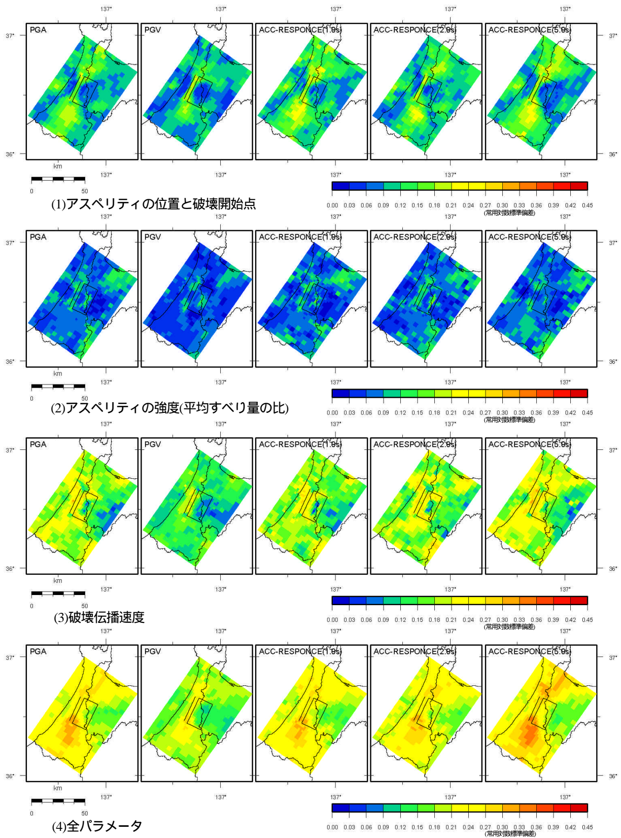
図 11 バラツキの対数標準偏差の空間分布(差分法)
