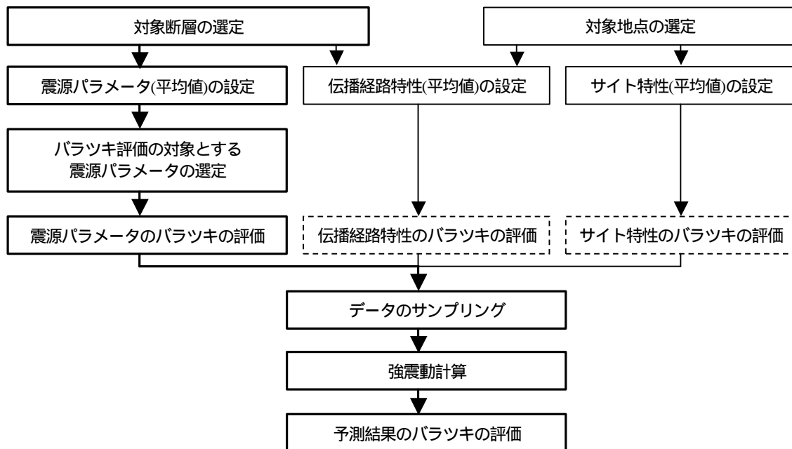
図1 強震動予測におけるバラツキ評価の流れ
