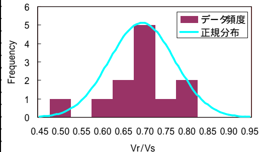
図2 破壊伝播速度のヒストグラム
