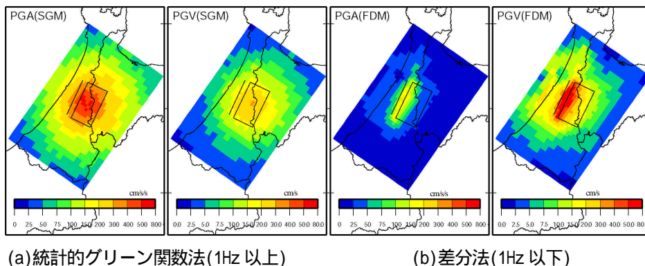
図9 PGA、PGV の平均値の空間分布
