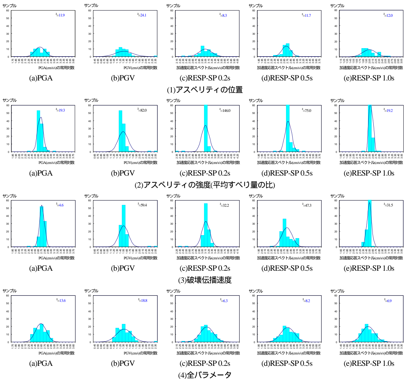
図7 強震動予測結果のヒストグラム(統計的グリーン関数法)
