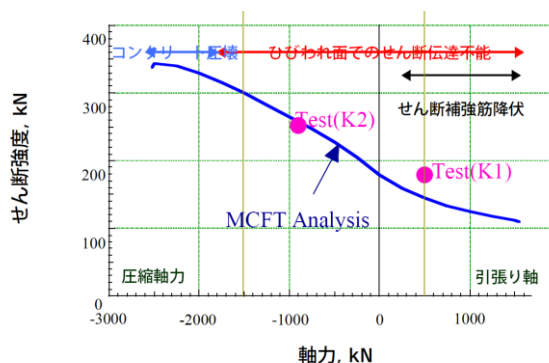
図 3.1.1-1 せん断強度と軸力との関係 (例)
