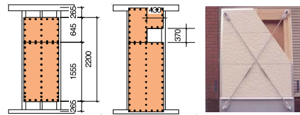
有開口面材耐力壁
